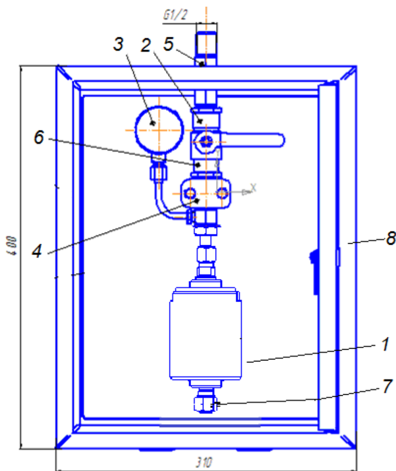
Рис. 1. Пост газоразборный ПГГ-65/35-з
